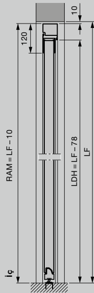
Alüminyum blok kasalı yan kapı, profil tipi 2 Açıklıkta montaj
