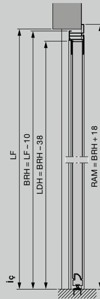
Alüminyum köşe kasalı yan kapı, profil tipi 2 Dıştan montaj
