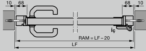
Alüminyum blok kasalı yan kapı, profil tipi 2 Açıklıkta montaj
