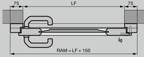
Masif ahşap yan kapı Açıklığın arkasına montaj
