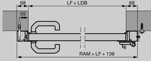
Alüminyum blok kasalı yan kapı, profil tipi 1 Açıklığın arkasına montaj
