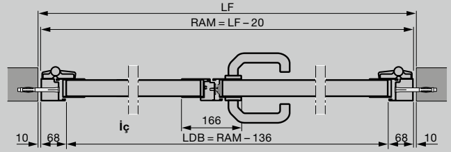
Alüminyum blok kasalı 2 kanatlı yan kapı, profil tipi 2 Açıklıkta montaj
