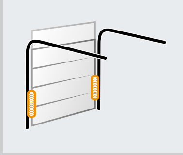
BZ kizak: Çekme yayı teknoloji ve eşgörünümlü kaplamalı çekme yay kızıağı
