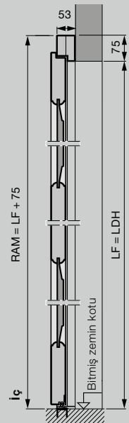
Masif ahşap yan kapı Açıklığın arkasına montaj
