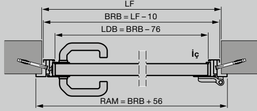
Alüminyum köşe kasalı yan kapı, profil tipi 1 veya 2 İç montaj
