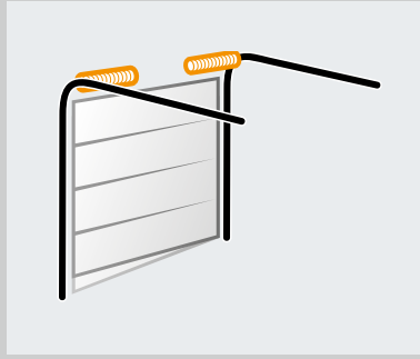
SN kizak: Eğimli alt panelli torsiyon yayı teknoloji normal kizak (maks. 300 mm yükseklik farkı)
