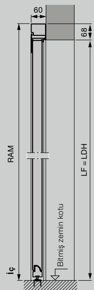
Alüminyum blok kasalı yan kapı, profil tipi 2 Açıklığın arkasına montaj
